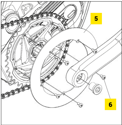
Copricatena
