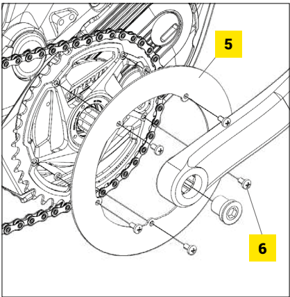
Kettenführung
