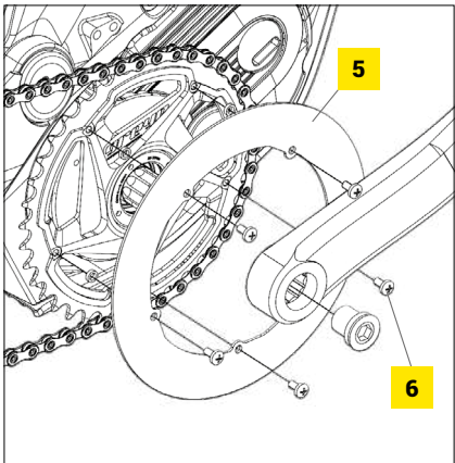
Chainguard
