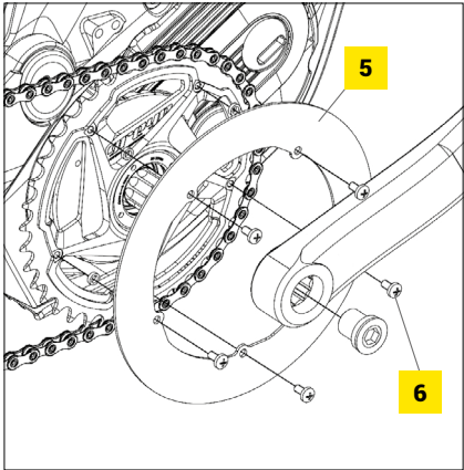
Copricatena
